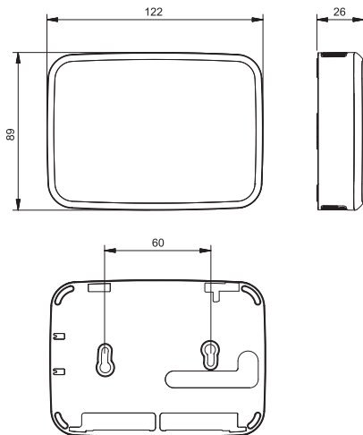
Fig.3: Dimensiones / Dimensions / Dimensioni / Abmessungen / Afmetingen / Rozměry
