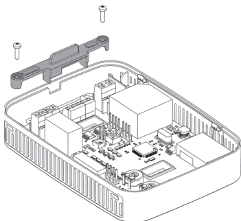
Fig.5: Retención cables / Cable retention / Fissaggio del cavo / Rétention de câbles / Zugentlastung / Kabel borging / Upevnění kabelů
