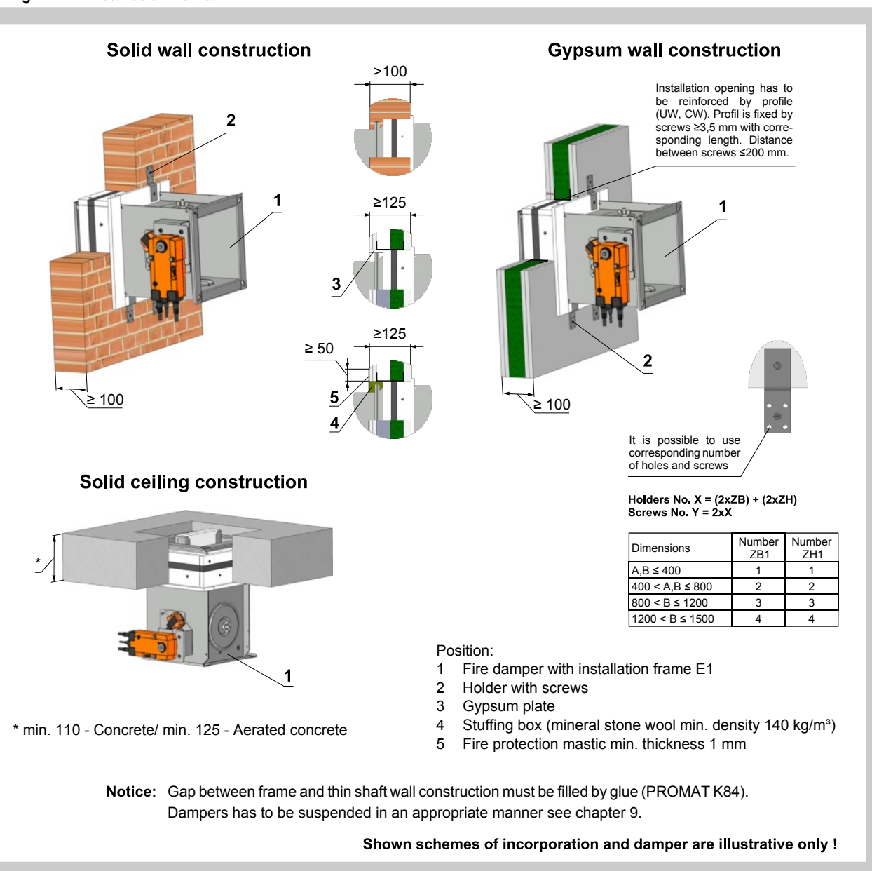
Fig. 72 Installation frame E1
