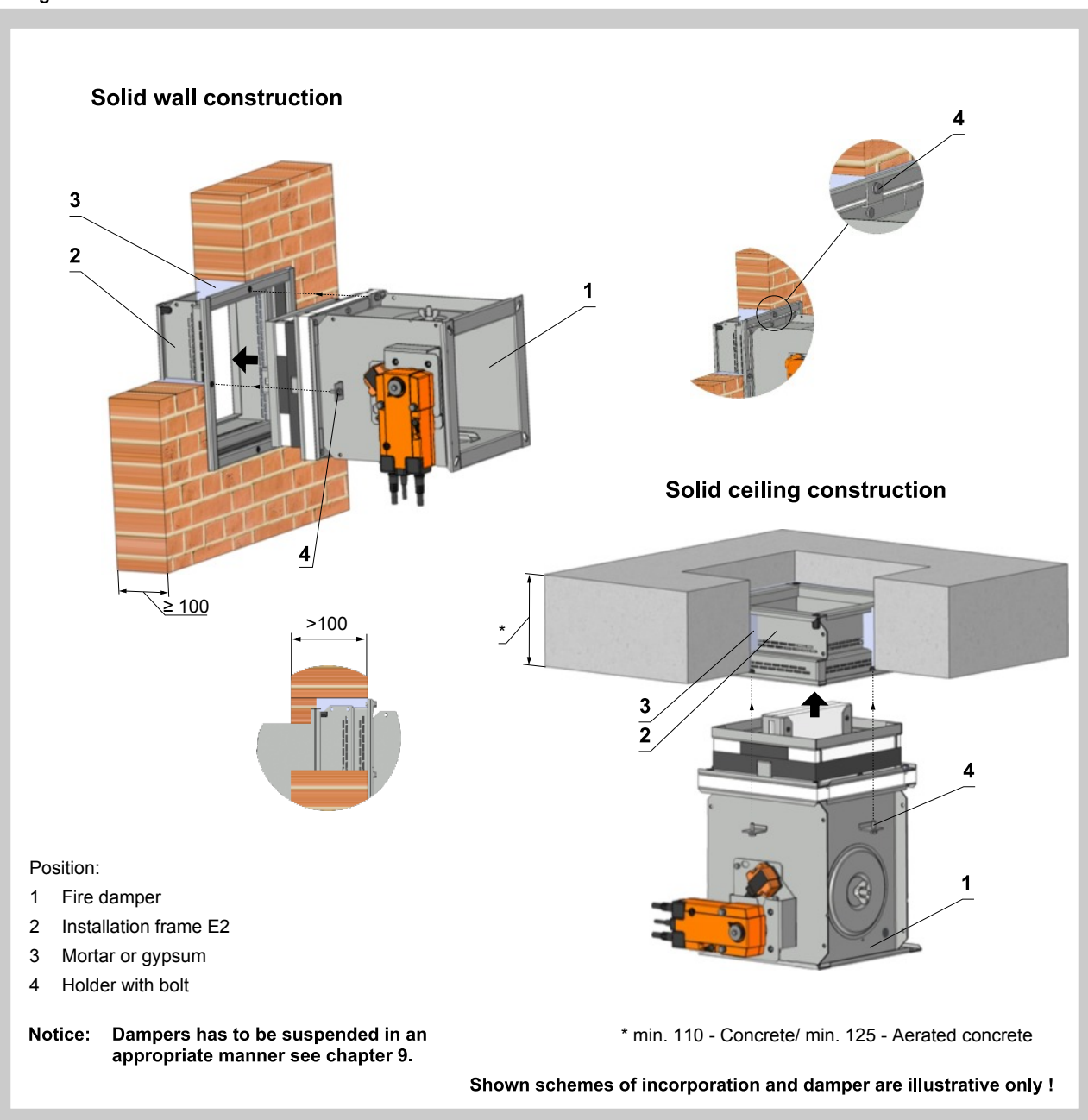
Fig. 73 Installation frame E2
