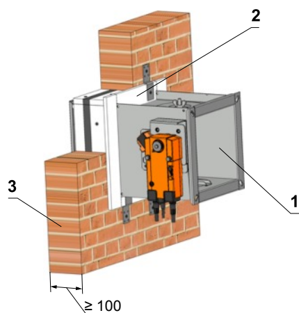
Installation frame E1
