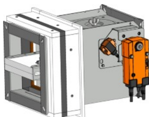
Installation frame E3
