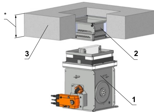
Installation frame E2
