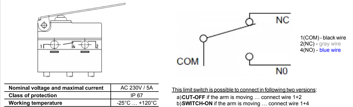
Fig. 6 Limit switch G905-300E03W1
