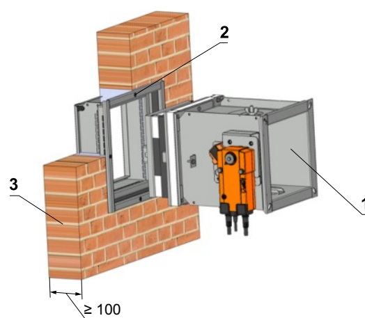
Installation frame E2
