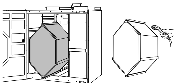
Obr. 4 Rekuperátor
