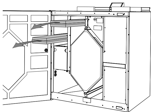
Obr. 3 Výměna filtrů
