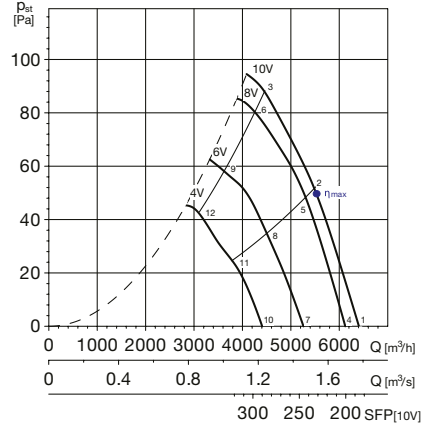
TXBR 450 Ecowatt
